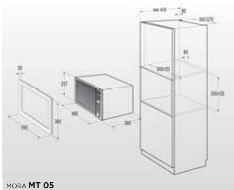
MORA MT 05
