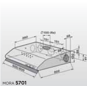
MORA 5701
