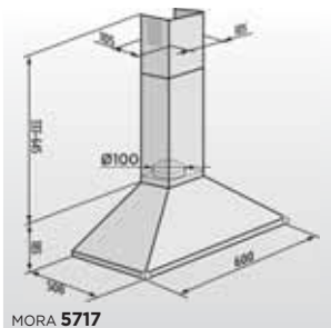
MORA 5717
