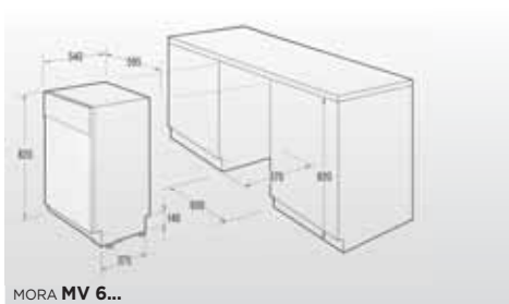
MORA MV 6...
