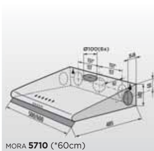
MORA 5710 (*60cm)
