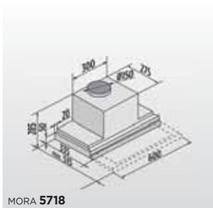
MORA 5718
