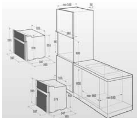
MORA MBO...
