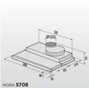
MORA 5708
