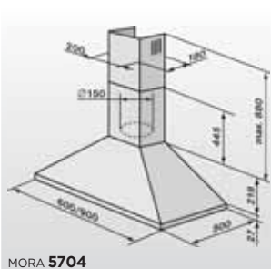
MORA 5704
